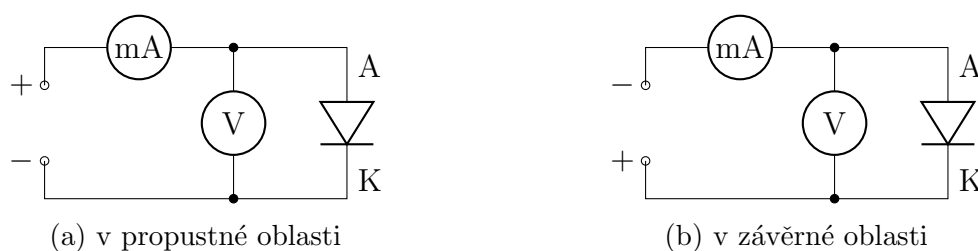
Schéma 1: Zapojení pro měření charakteristiky diody
